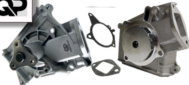
Bomba de Agua Mazda B3/5/6/323 Festiva Turpial
