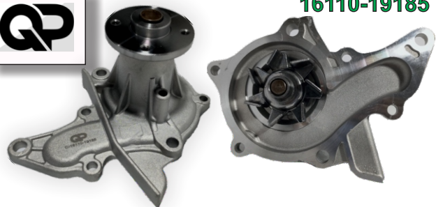
Bomba de Agua Toyota Corolla 1.8 L4 1993-97 Cekica 1994-97 JS-T147 86A
